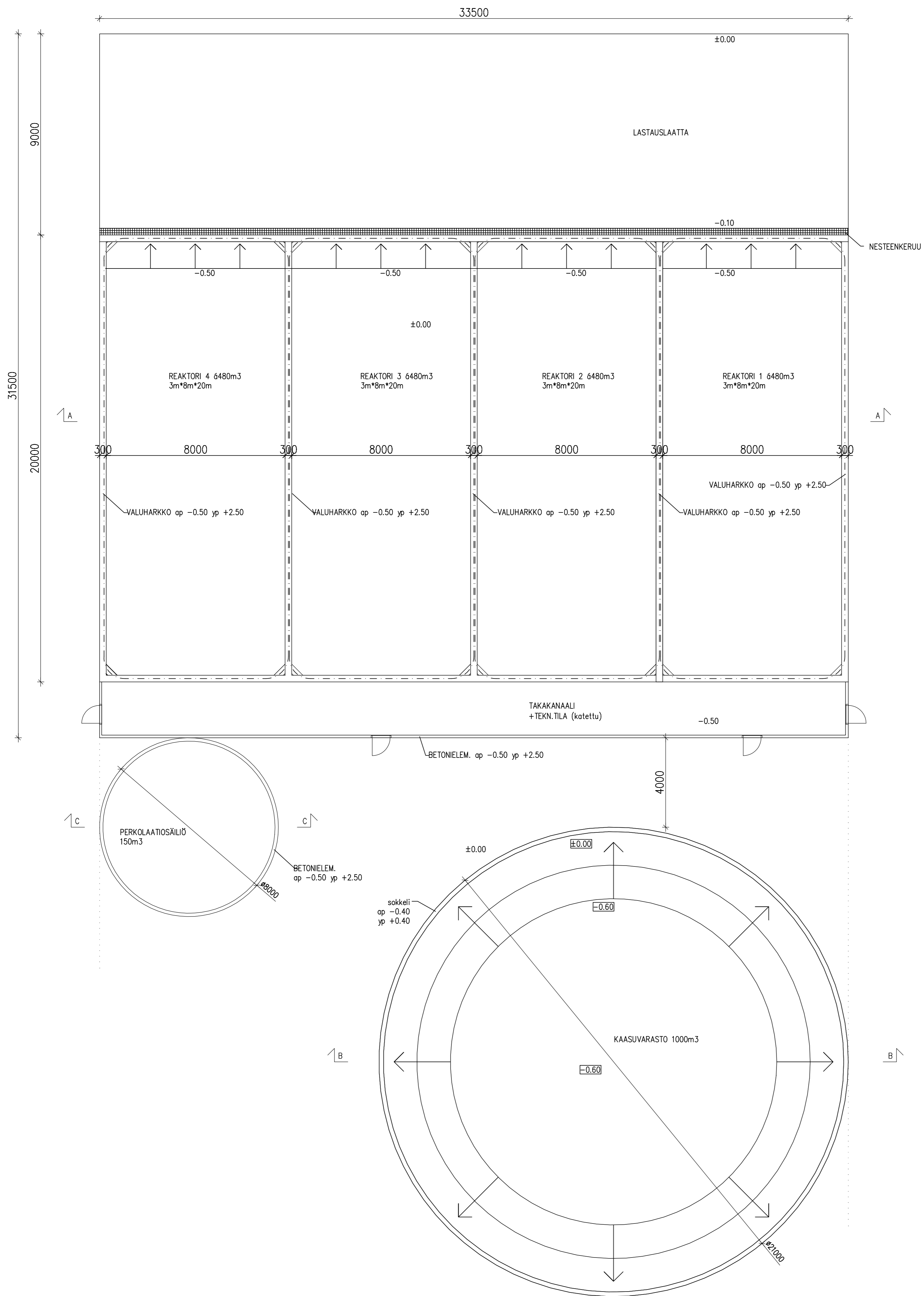
REAKTORIT, KAASUVARASTO JA PERKOLAATIOSÄILIÖ POHJAPIIRROS 1:100
