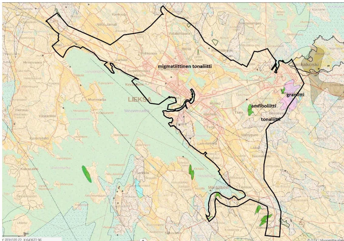
Kuva 2. Alueen kallioperä (gtk.fi/maankamara).
